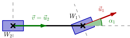
Abbildung 2. Einspurmodell aus der Fahrdynamik
