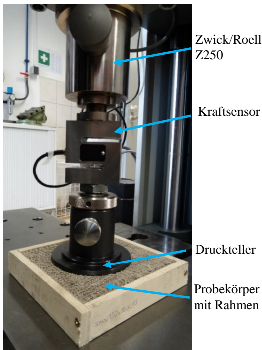
Abbildung 7. Versuchsaufbau zur Ermittlung des Kraft-Verformungsverlaufs verdichteter sinuswabenförmiger Pappwerkstoffe
