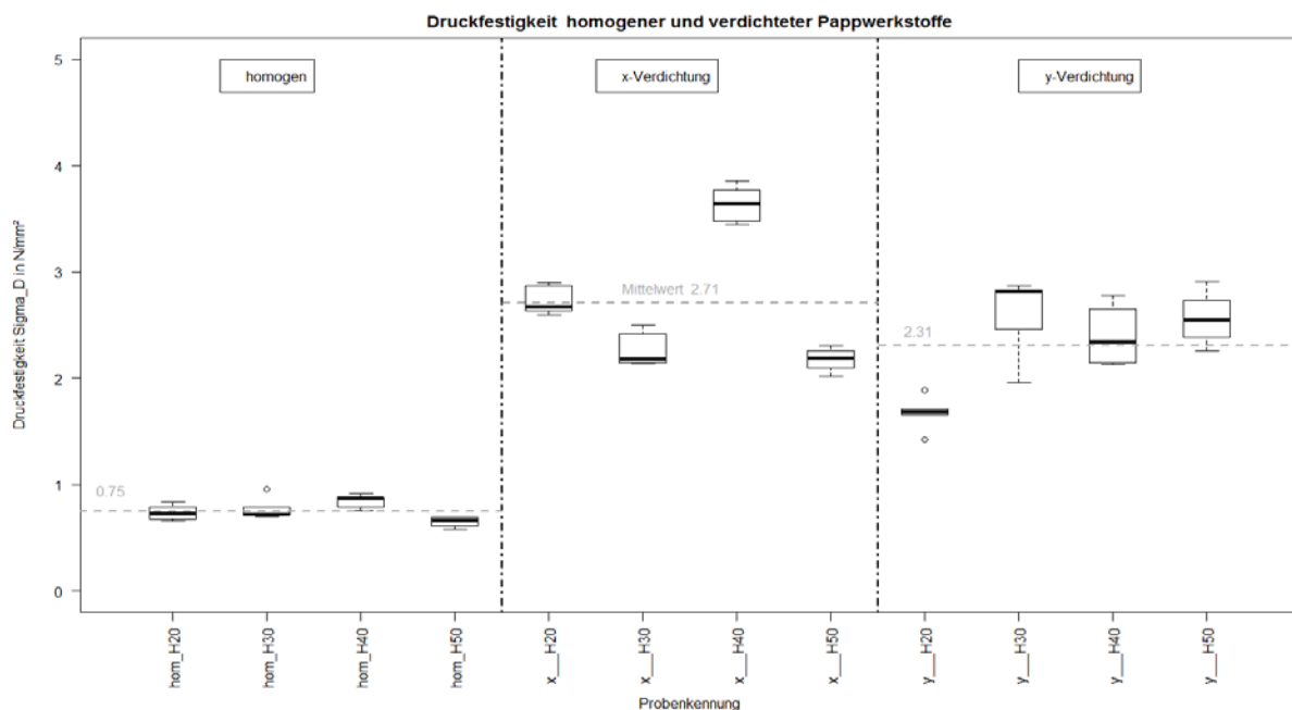
Abbildung 9. Boxplots der ermittelten Druckfestigkeit homogener und verdichteter sinuswabenförmiger Pappwerkstoffe
