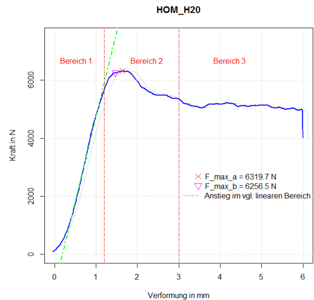
Abbildung 8. Charakteristische Kraft-Verformungs-Kurve eines Druckversuchs von sinuswabenförmigen Pappwerkstoffen
