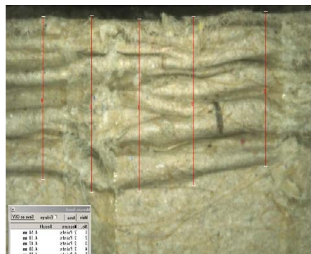
Abbildung 10. Verformungsverhalten eines unverdichteten Pappwerkstoffes hom_H20 (Mikroskopie)
