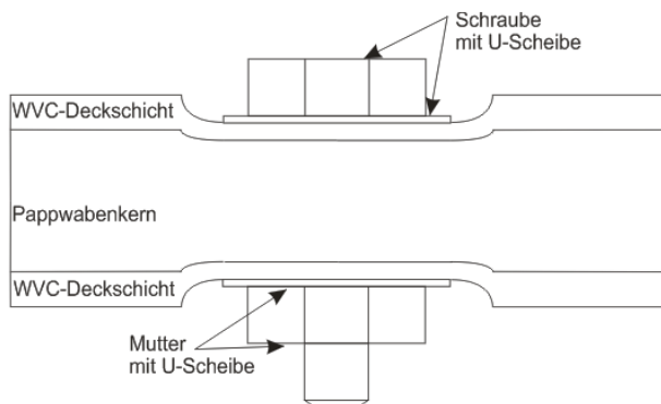
Abbildung 2. Schraubverbindung in Sandwichelement nach dem Spannen mit Verformung der Deckschicht und des Kerns
