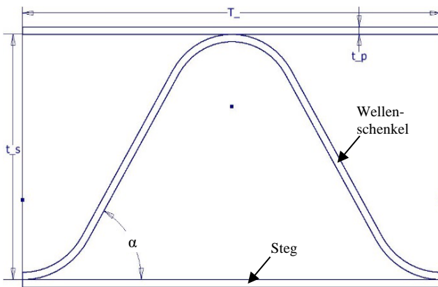
Abbildung 4. Geometrie und Parameter einer Welle innerhalb des homogenen sinuswabenförmigen Pappwerkstoffes
