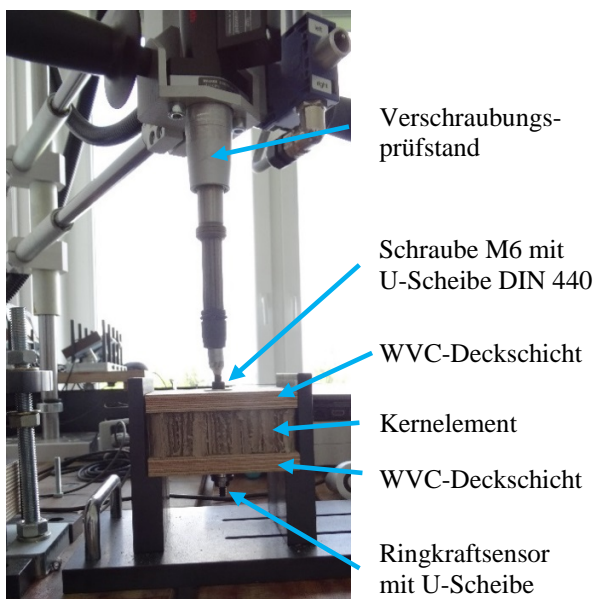
Abbildung 12. Versuchsaufbau zur Untersuchung von Schraubverbindungen in Sandwichelementen
