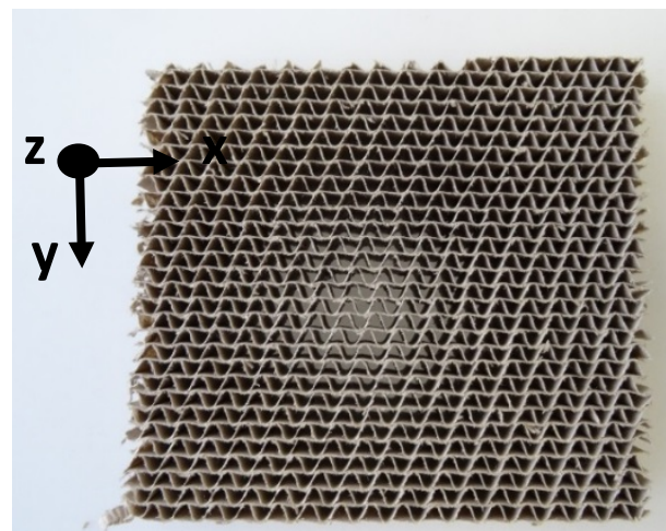
Abbildung 3. Ansicht von oben (z-Richtung, senkrecht zur Plattenebene = x-y Ebene) auf den unverdichteten, homogenen sinuswabenförmigen Pappwerkstoff
