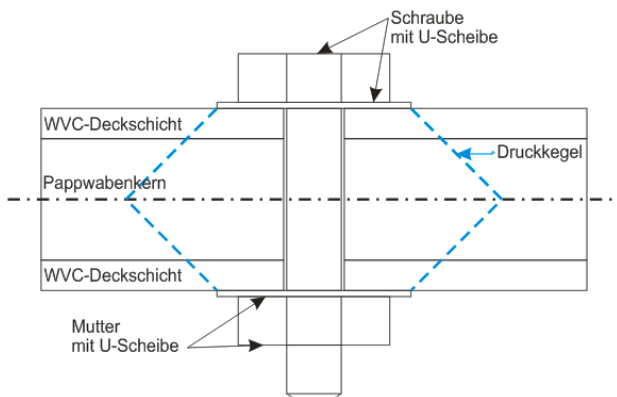
Abbildung 1. Schraubverbindung mit möglichem Druckkegel (blaue Strichlinie) in Sandwichelement vor dem Spannen der Schraube [4]
