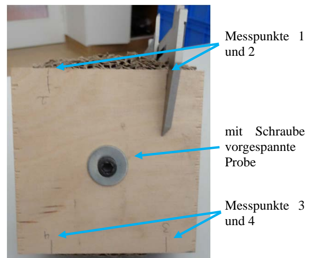
Abbildung 13. Messprinzip zur Bestimmung der Dicke der un-/ verschraubten Sandwichelemente
